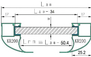
Вставка из стекла (зеркала) 4мм
