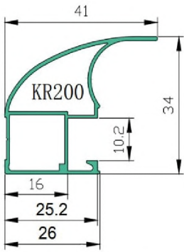
Вставка из ДСП 10мм
