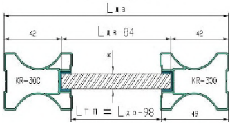
Вставка из стекла (зеркала) 4мм
