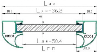
Вставка из стекла (зеркала) 4мм
