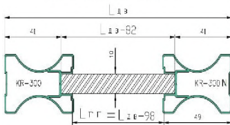
Вставка из ДСП 8мм
